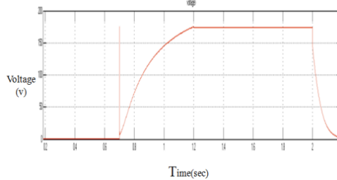
Fig. 7. voltage o a supercapacitor.
