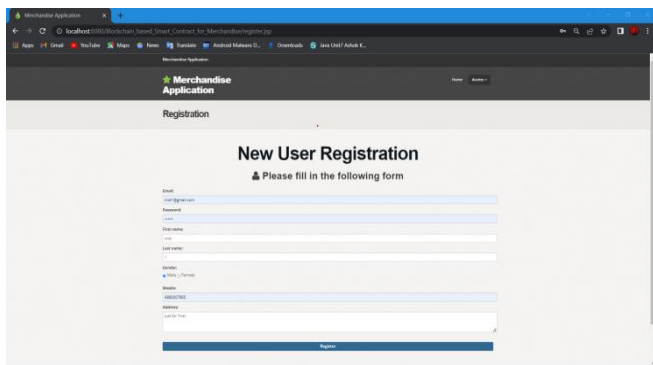
Fig. 7. Register Page
